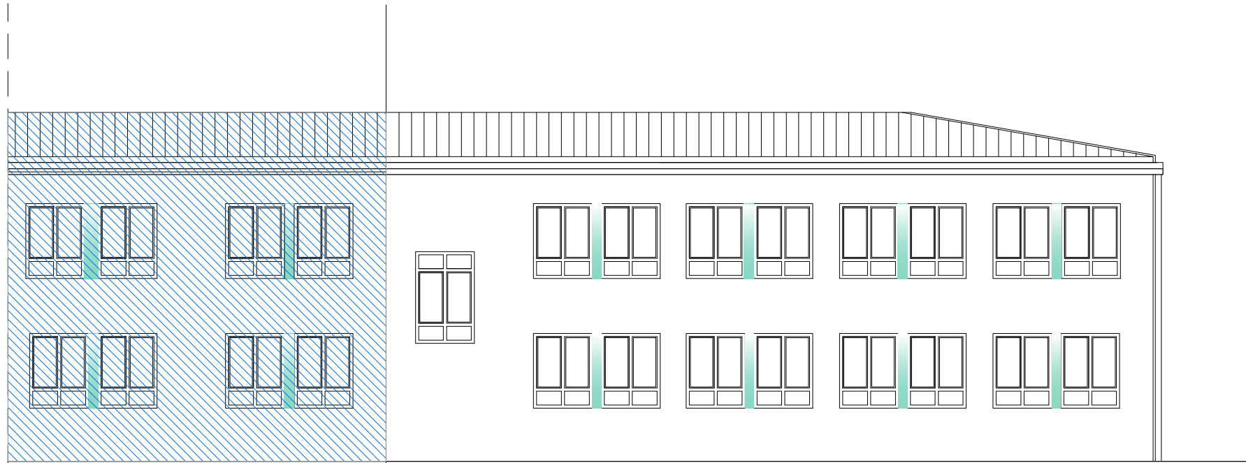
FASADA VZHOD
